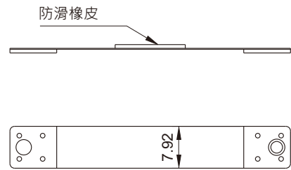
固定鋼帶尺寸圖
